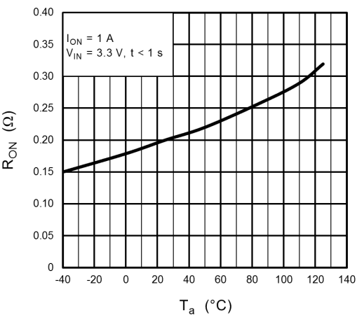
Fig. 12.4 R_{ON} - T_a
