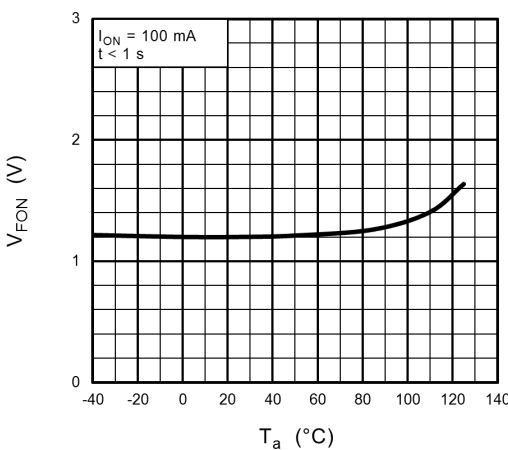
Fig. 12.5 V_{FON} - T_a
