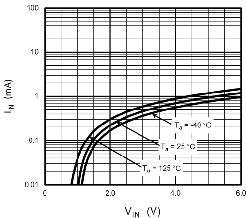
Fig. 12.1 I_{IN} - V_{IN}
