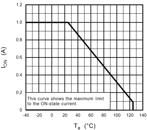
Fig. 12.2 I_{ON} - T_a
