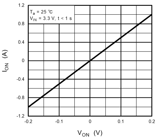
Fig. 12.3 I_{ON} - V_{ON}
