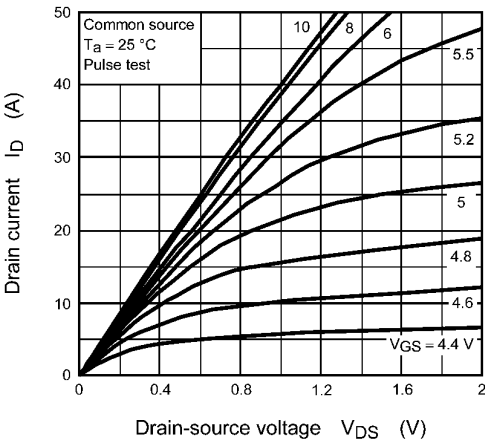
Fig. 8.2 I_D - V_{DS}
