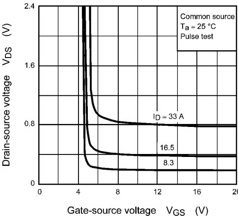
Fig. 8.4 V_{DS} - V_{GS}
