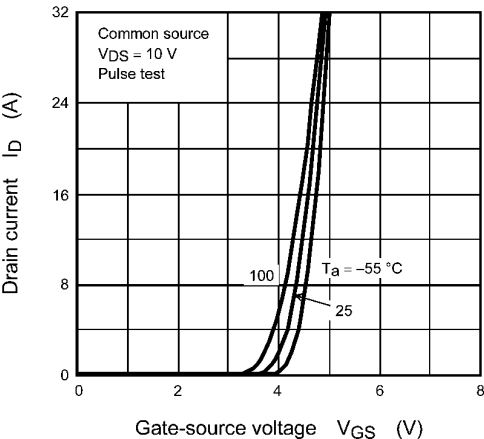
Fig. 8.3 I_D - V_{GS}
