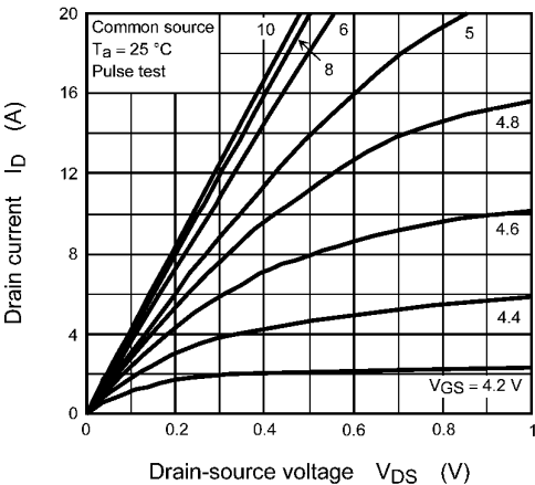
Fig. 8.1 I_D - V_{DS}
