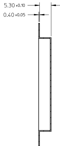
SECTION V-V
