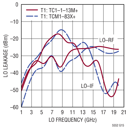
LO Leakage
