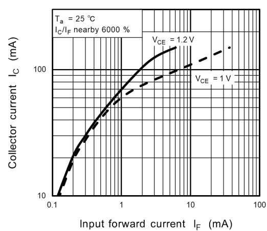
Fig. 12.10 I_C - I_F
