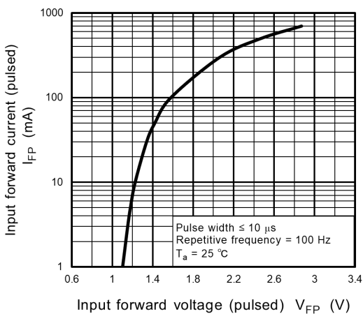
Fig. 12.6 I_{FP} - V_{FP}
