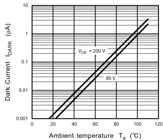
Fig. 12.8 I_{\text{DARK}} - T_a
