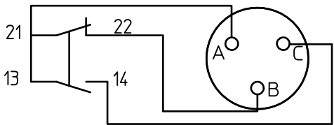
Schaltbild:
