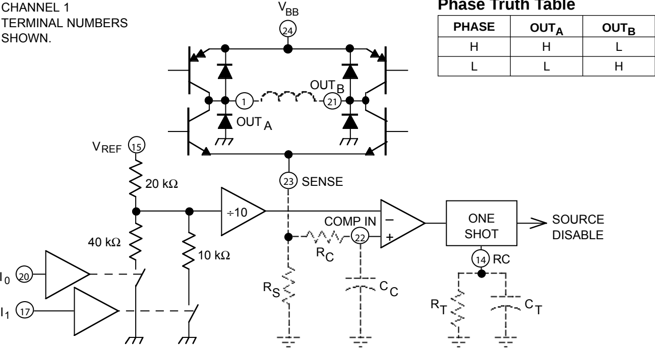
Dwg. EP-007-5
