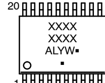
TSSOP-20
