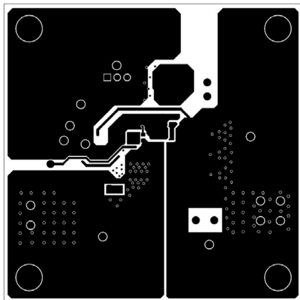
Fig. 6: Bottom
