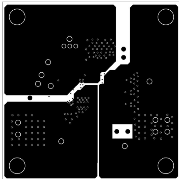
Fig. 8: Layer 3, VCC1
