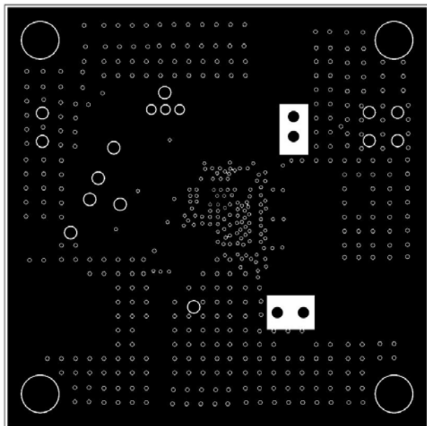
Fig. 7: Layer 2, GND 1
