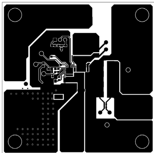
Fig. 5: Top
