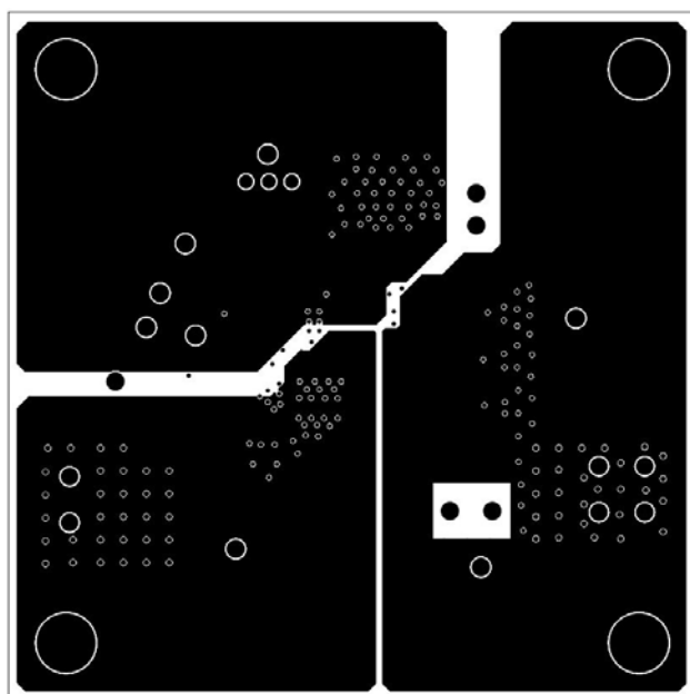
Fig. 10: Layer 5, VCC2
