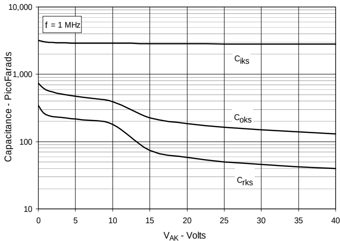
Fig. 5. Capacitance
