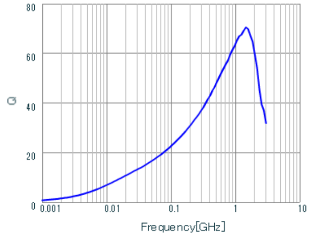
LQW15AN30NG80 Q.
