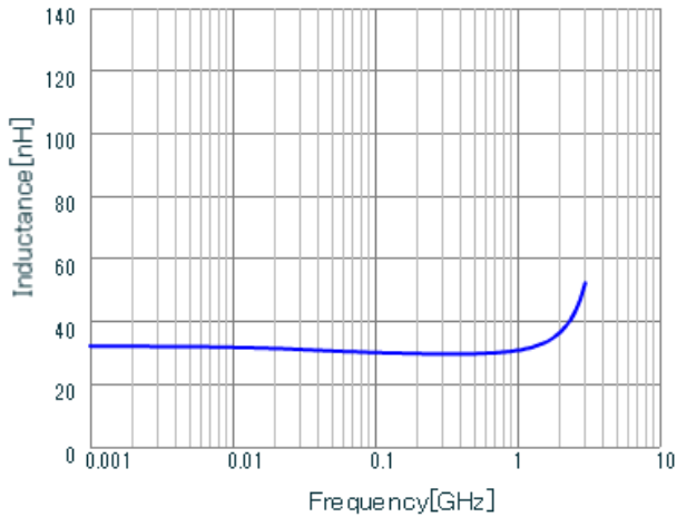
LQW15AN30NG80 L.
