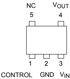
ESV(SOT-553)
