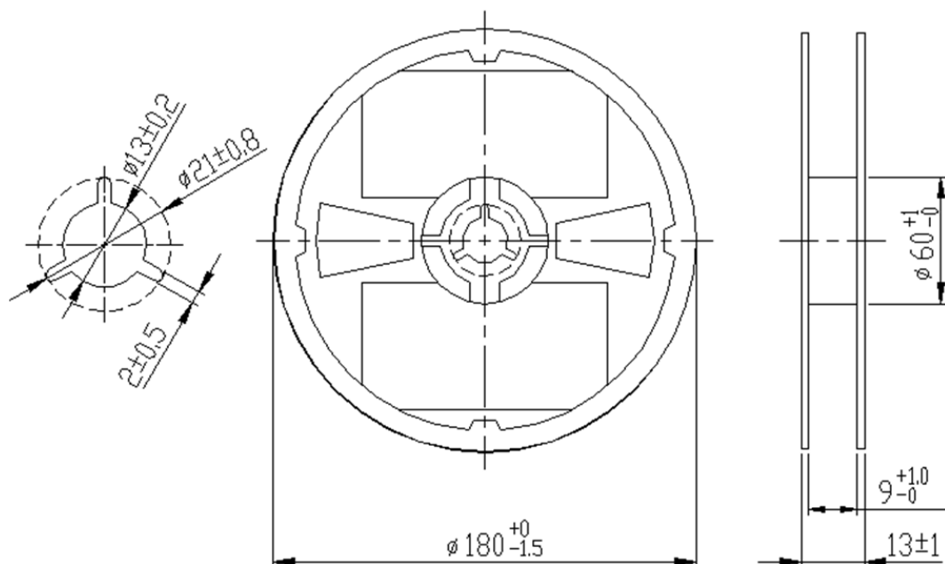
Reel Dimensions
