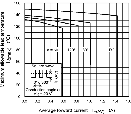
Fig. 10.4 T_{l(max)} - I_{F(AV)}
