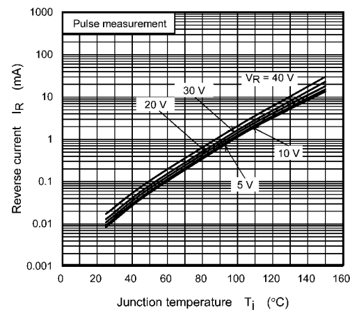
Fig. 10.8 I_R - T_j
