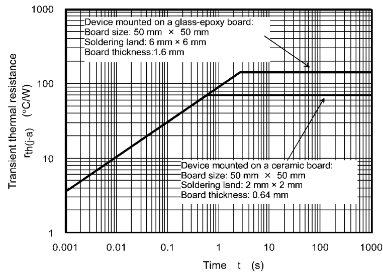
Fig. 10.6 r_{th(j-a)} - t
