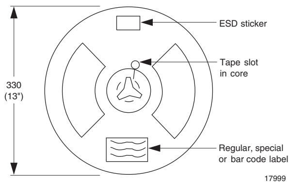
Fig. 18 - Reel Dimensions
