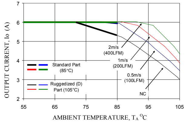
V_o = 1.2V
