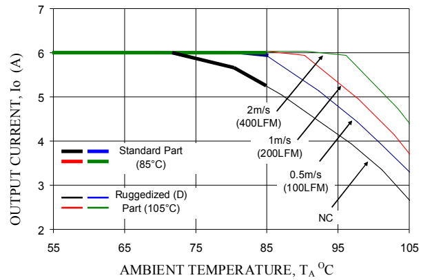
V_o = 2.5V
