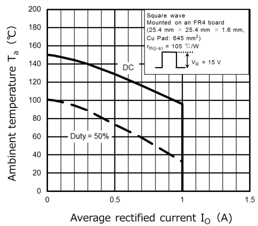
Fig. 9.6 T_a - I_O
