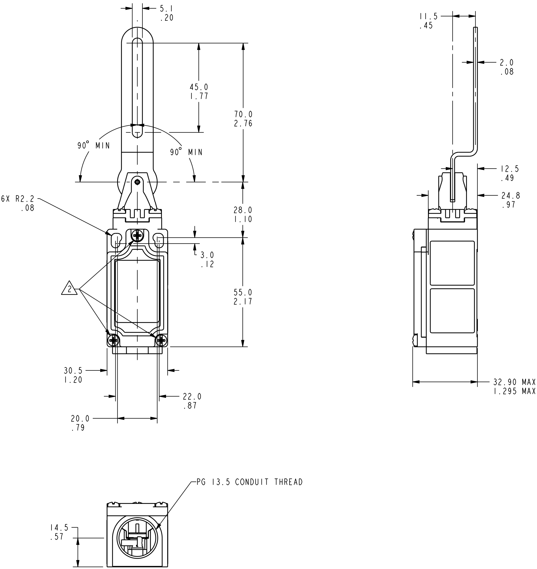
ACTUATOR CODE 2
