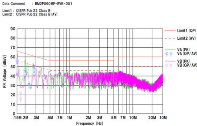
Figure 23. V_{IN} : 115 Vac / 60 Hz, I_{OUT} : 1.67 A
