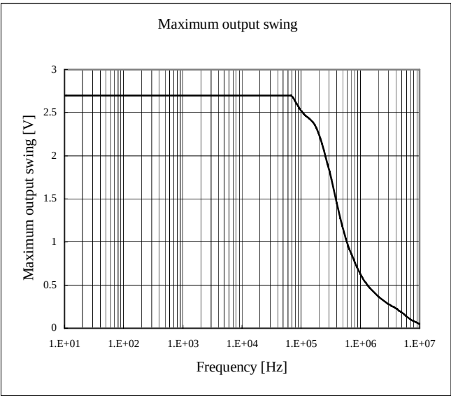
□ Maximum output swing vs. Frequency (VDD=2.7V, Ta=25°C, Av = 1, RL = 10kΩ)
