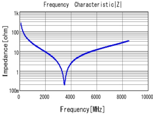
■ GCQ1555C1H6R0DB01 |Z| DC0V, 25degC
