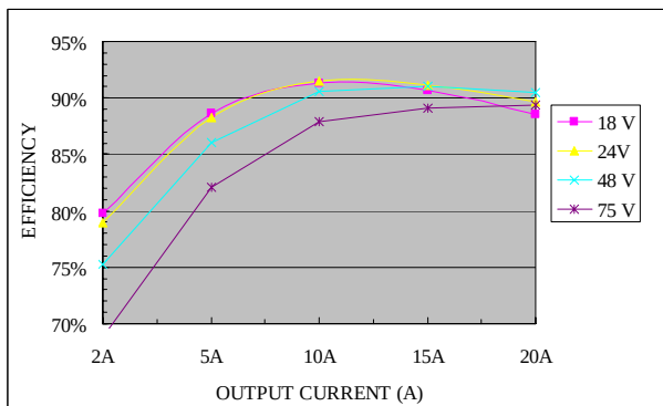
Vo=5.0 V
