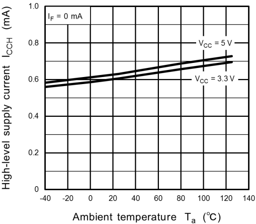
Fig. 13.2.8 I_{CCH} - T_a
