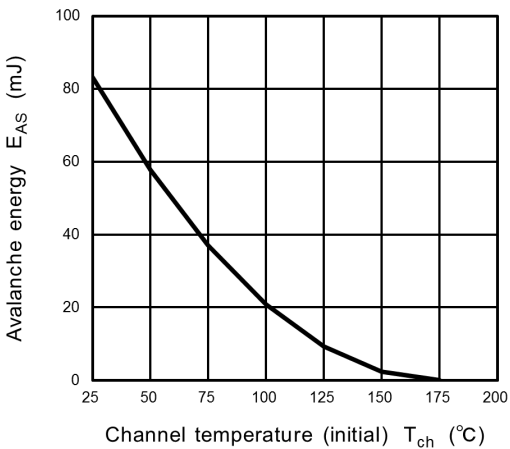
Fig. 8.15 E_{AS} - T_{ch}
