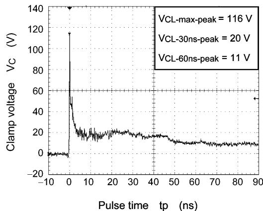
Fig. 6.1.1 +8 kV
