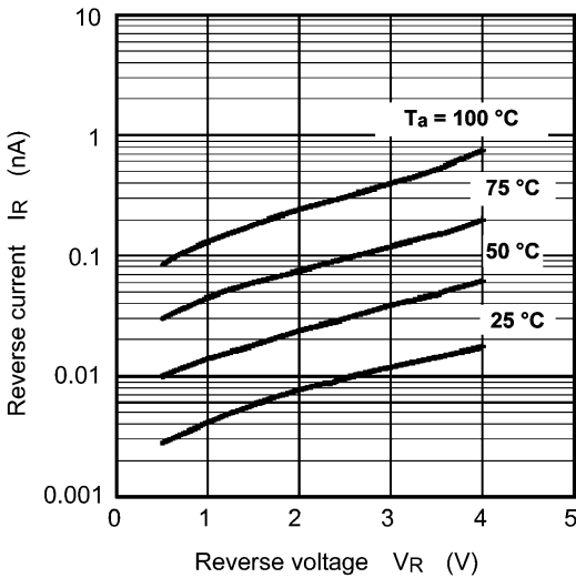
Fig. 9.2 I_R - V_R
