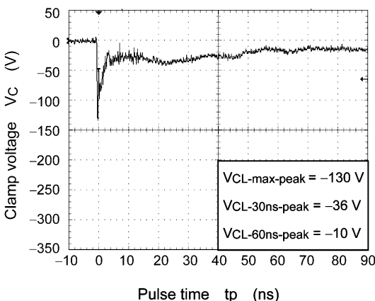
Fig. 6.1.4 -15 kV
