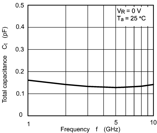
Fig. 9.4 C_t - f
