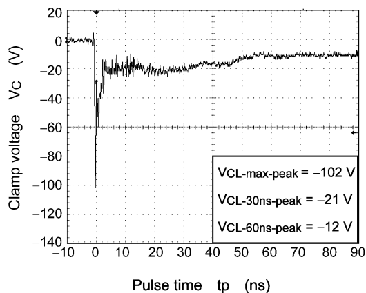
Fig. 6.1.2 -8 kV
