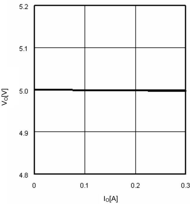
Fig.13 Io-V O
