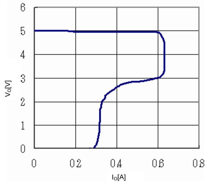
Fig.17 OCP
