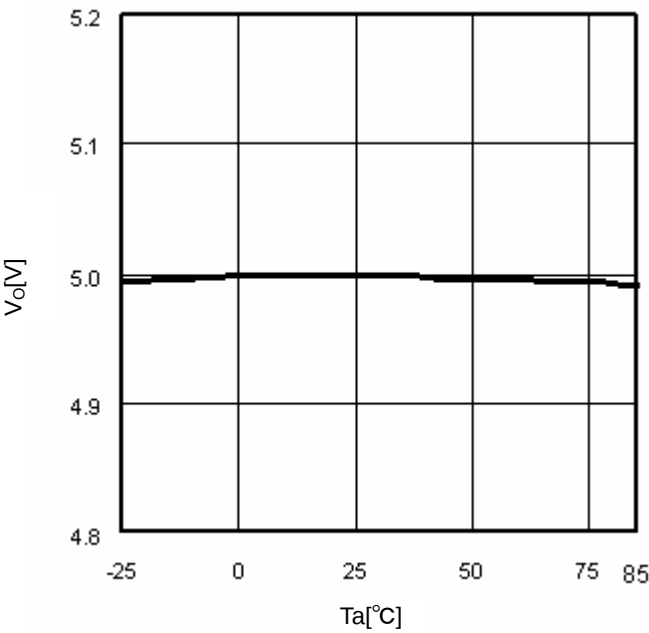
Fig.9 Ta-Vo (Io=0mA)
