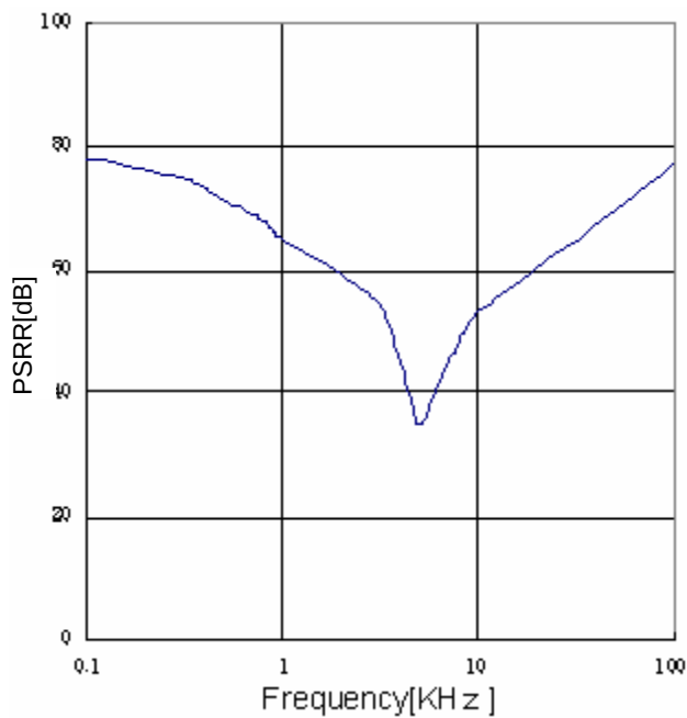
Fig.21 PSRR( I_o=0 mA)
