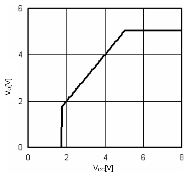
Fig.15 V_{CC}-V_O ( I_O=0\text{mA} )
