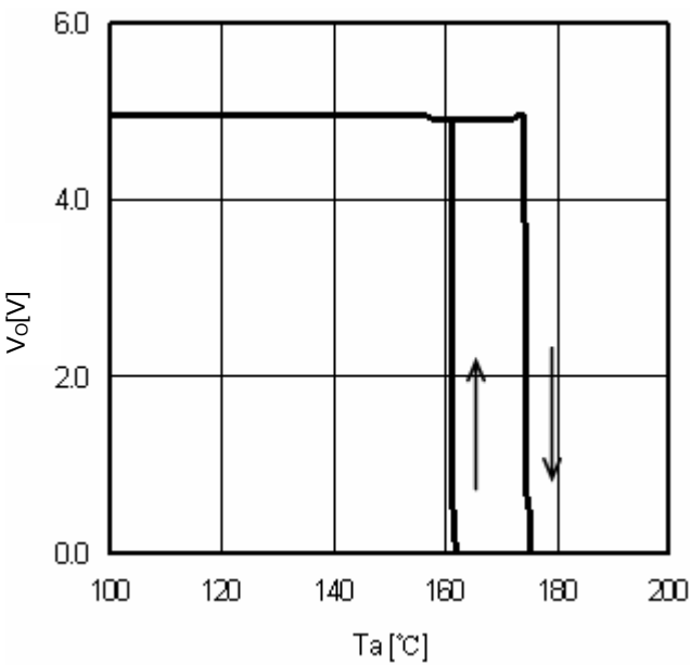
Fig.16 TSD ( I_O=0\text{mA} )
