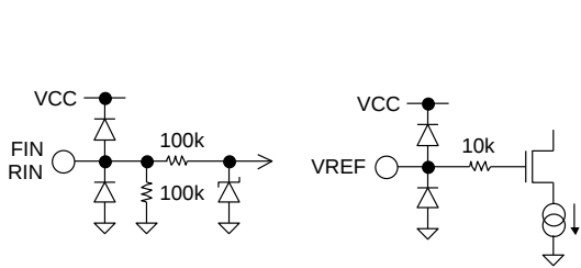
Figure 40. FIN / RIN
