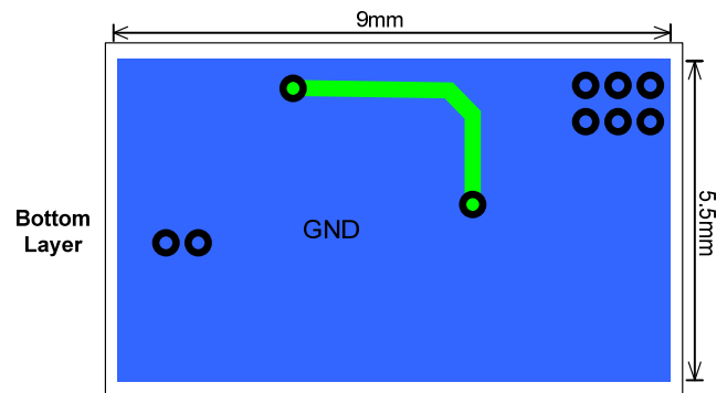
Figure 4— Bottom Layer
