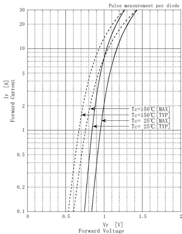
UD8KBA80 Forward Voltage
