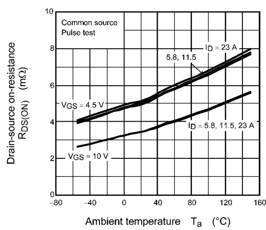
Fig. 8.6 RDS(ON) - Ta
