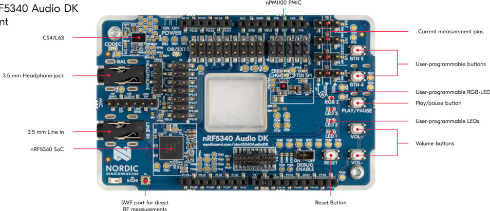
nRF5340 Audio DK back
