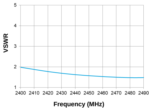
2.4 GHz VSWR
