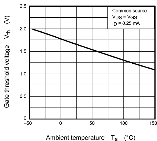
Fig. 7.6 V_{th} - T_a
