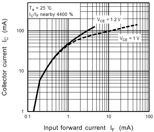
Fig. 11.10 I_C - I_F
