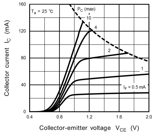
Fig. 11.7 I_C - V_{CE}
