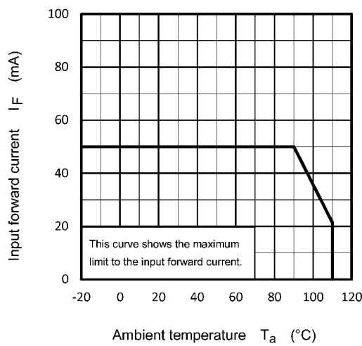
Fig. 11.1 I_F - T_a
