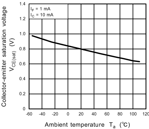
Fig. 11.9 V_{CE(sat)} - T_a
