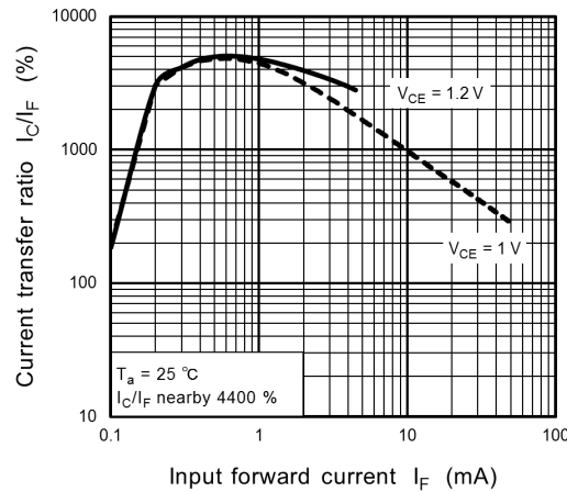
Fig. 11.11 I_C/I_F - I_F
