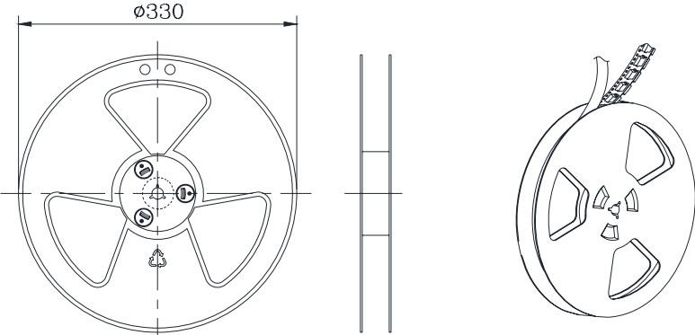
1 Reel : 1000PCS
