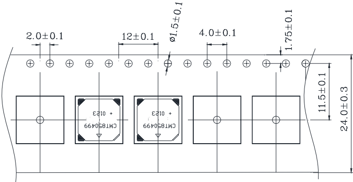
1 Reel : 1000PCS
