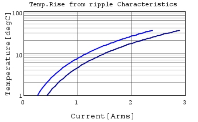
GRM155R61E105MA12 Temp.rise — 500kHz —
