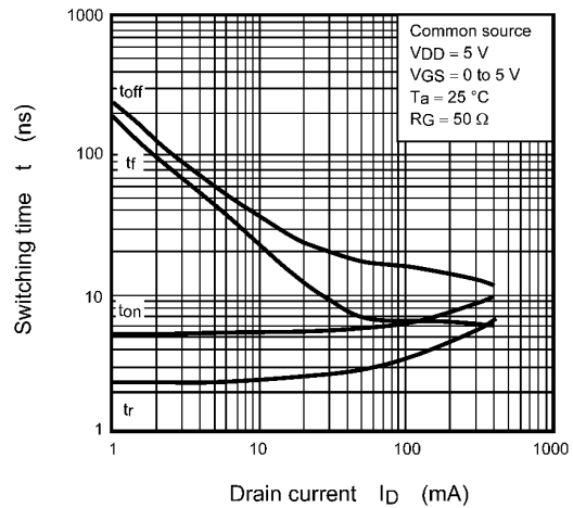
Fig. 8.10 t - I_D
