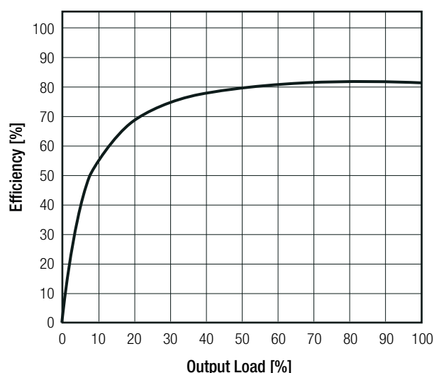
R2SX-0505S(/H)
