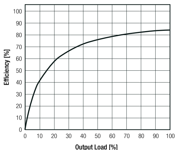
R2SX-2424S(/H)
