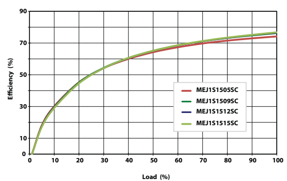
15V Input
