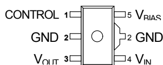
NJM2842U2
