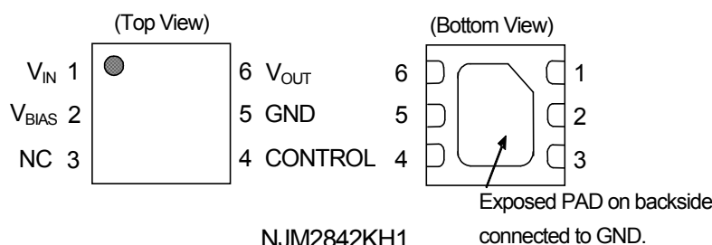
NJM2842KH1
