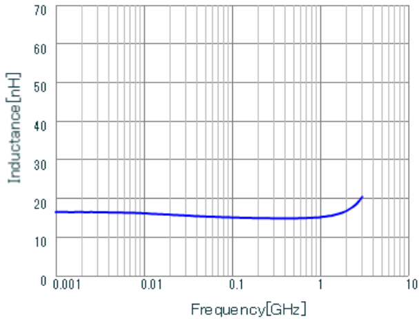
LQW15AN15NG8Z L.
