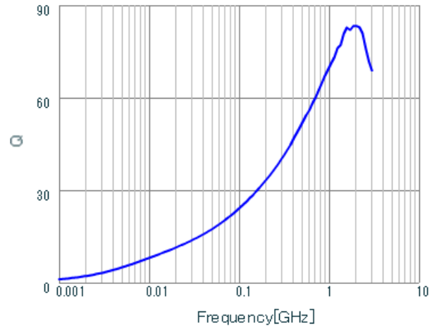
LQW15AN15NG8Z Q.
