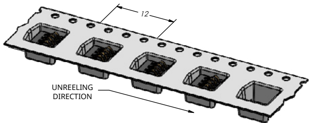
PACKAGING PER EIA-481 1,100 PARTS PER 330 mm REEL
