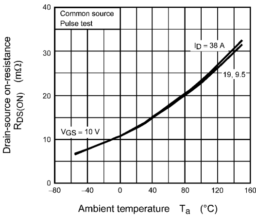
Fig. 8.9 R_{DS(ON)} - T_a
