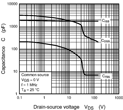
Fig. 8.11 Capacitance - V_{DS}
