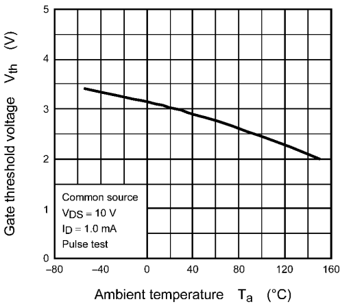
Fig. 8.8 V_{th} - T_a
