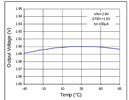
Fig 86. VOUT - Temp
