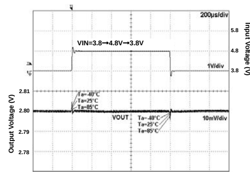
Fig 206. VIN Response
