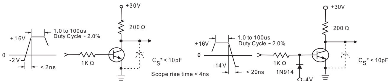
Fig. 1 Turn-On Time
