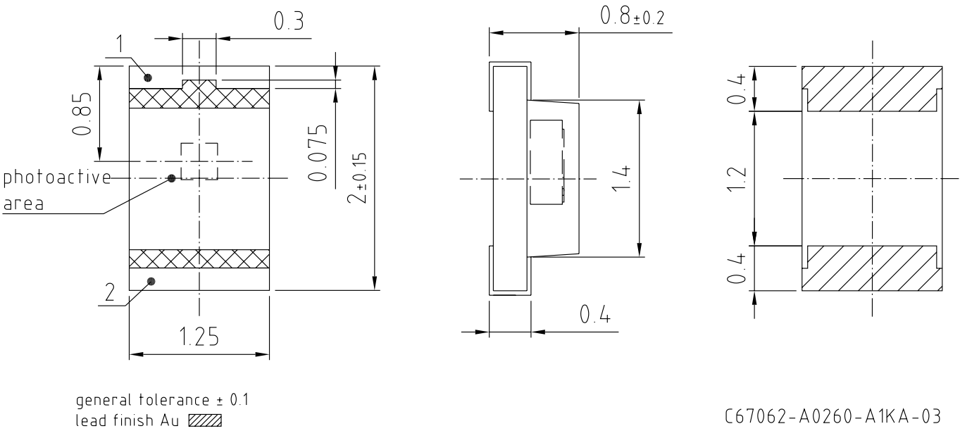
尺寸图 3)
