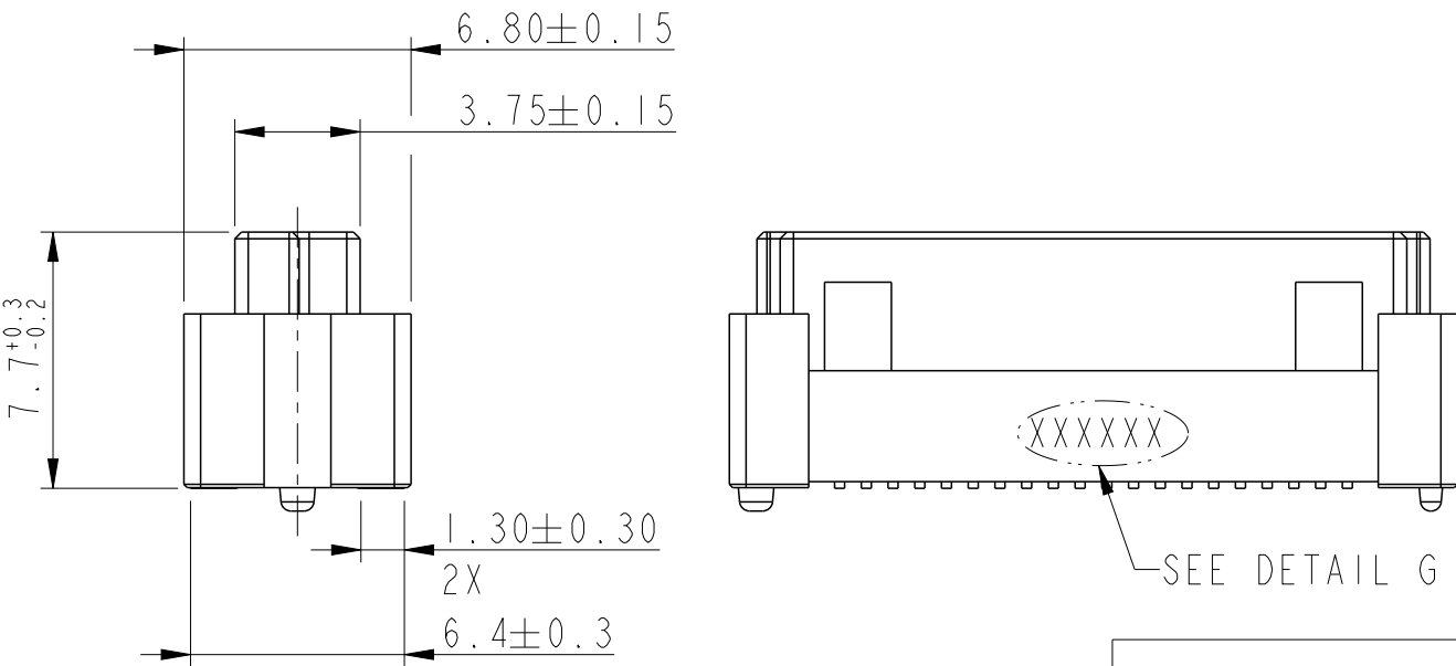
RECEPTACLE 2
