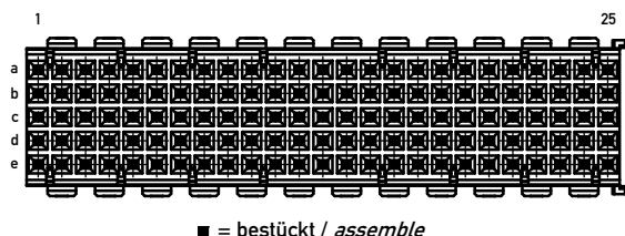
Bestückungsplan / Contact layout
