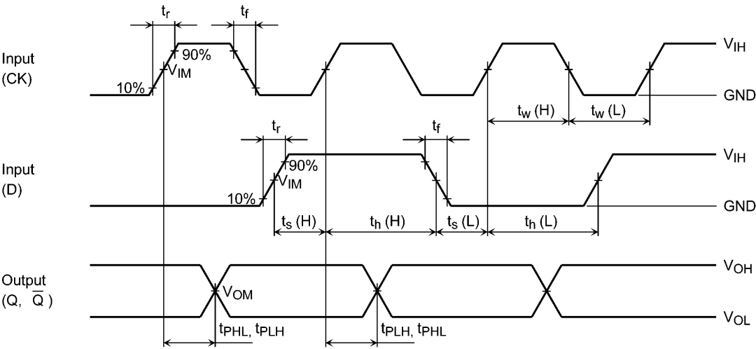
Fig. 11.8.1 t_{PLH} , t_{PHL} , t_w , t_s , t_h
