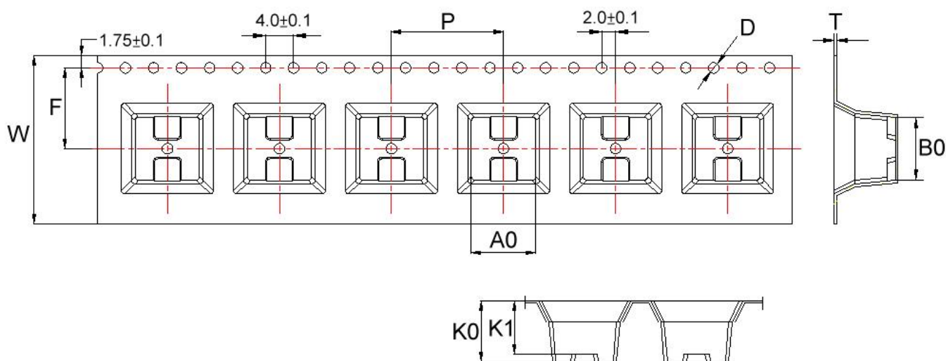
Reel Dimensions
